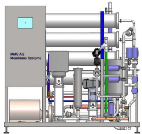
BeerMAX 120 Frontansicht
