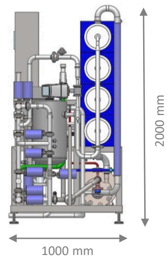
BeerMAX 120 Seitenansicht
